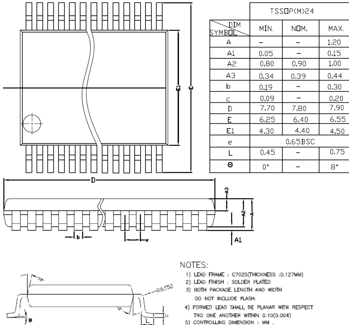
图 29 TSSOP24 封装图
