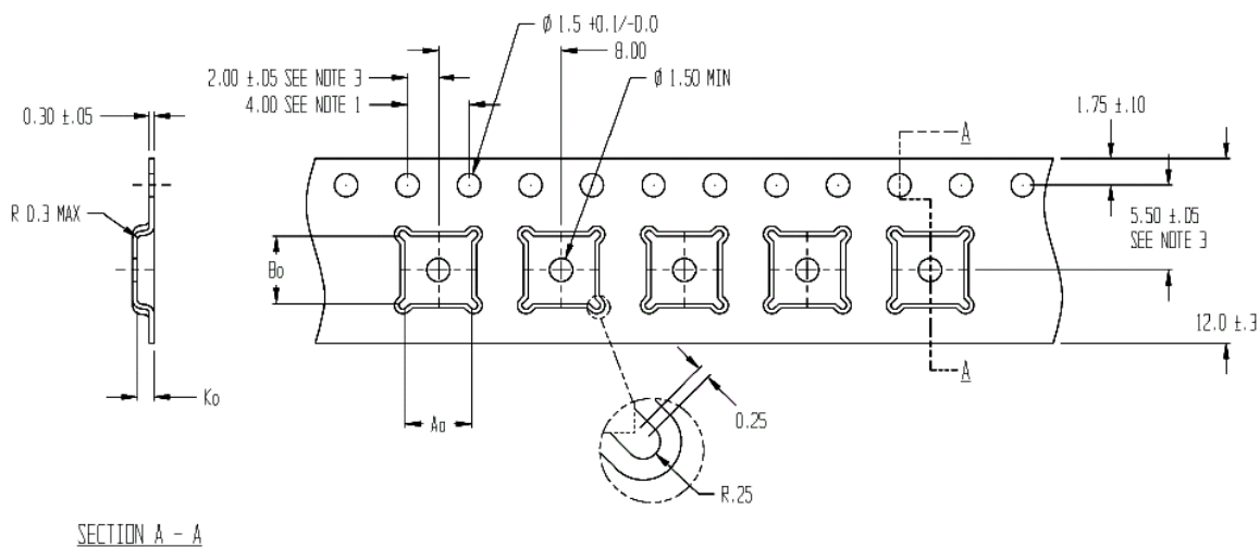
图 30 包装带尺寸
